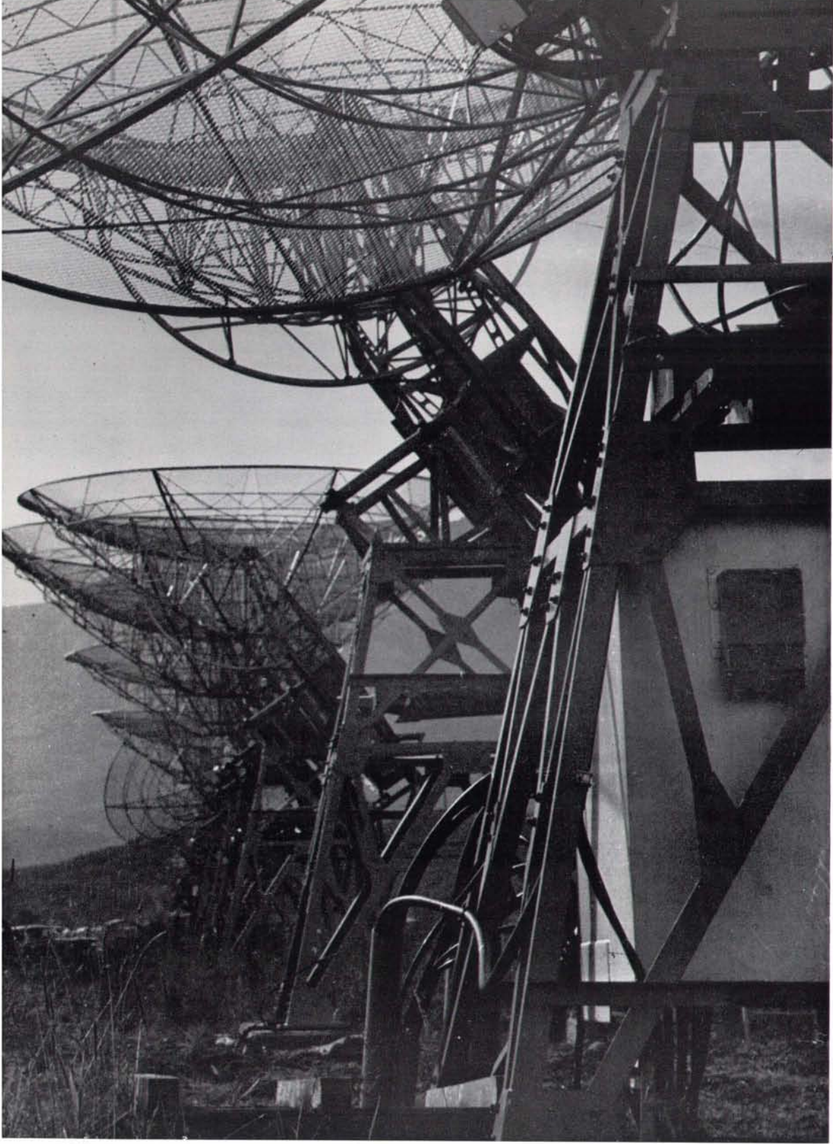
▲160 MHz 太陽電波干渉計のアンテナ群。アンテナの直径は6メートルある
