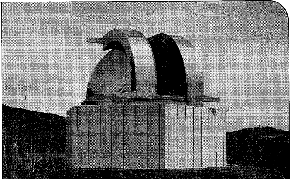
東京大学鹿儿岛宇宙空間観測所 φ6.5m天体観測室ドーム
