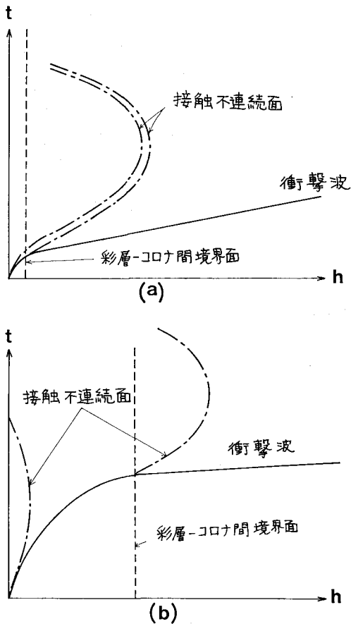
図3 ジェットの流体力学的構造の模式図。(a) ショック・チューブ型, (b) クレスト・ショック型。
