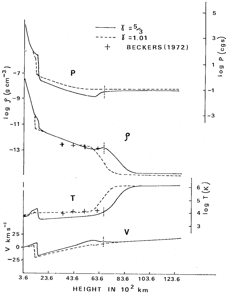
図2 数値実験(実線及び点線)とスピキュールの観測(+ )の比較。γは比熱比である。
