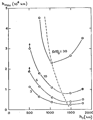
図5 h_0 の関数として示したジェットの高さ ( h_{max} ).
