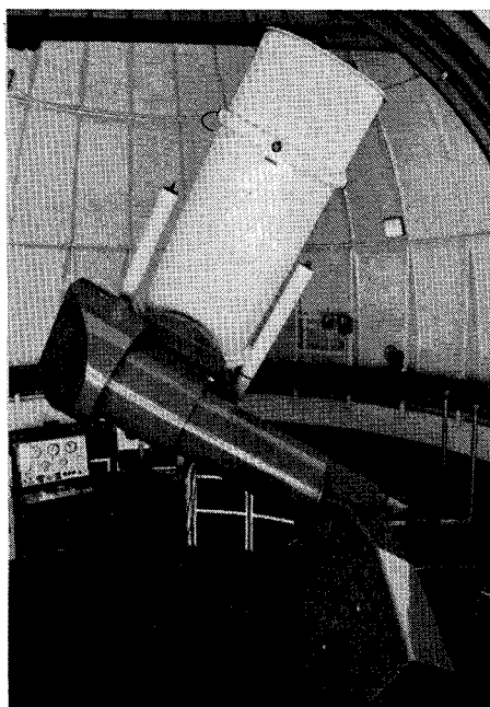
SWOPE 1m TELESCOPE (Las Campanas 天文台)
