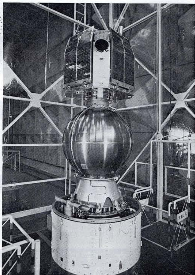
▶ 3段目球形モーターにとりつけられた「てんま」
