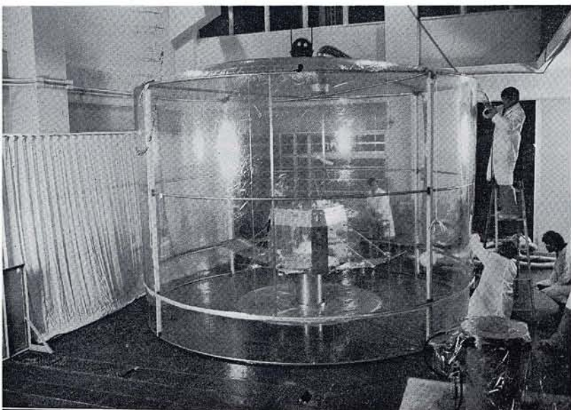
◀ 慣性能率の測定 全体をヘリウム中に入れて行う
