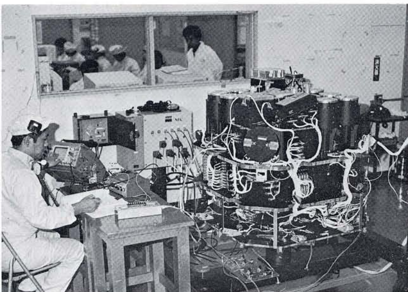
◀ 観測機器の動作チェック
