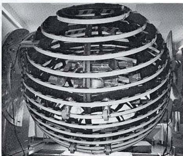
衛星の磁気モーメント測定 ▶
