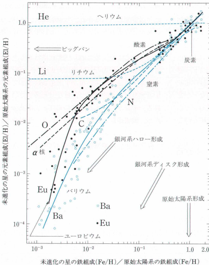
図1 横軸の鉄組成 (=Fe/H) で代表される物質進化に応じて、縦軸に各元素の組成 (=E/H) がどのように進化したかを示す。但し、横、縦軸共に原始太陽系の組成に対する相対値で示されている。これは、古い星を含む多数の星(その表面化学組成が誕生時の星間物質の化学組成を保存しているさまざまな年齢の主として未進化の星)の化学分析から得られた結果を数個の元素について模式的に示したものである( \alpha 核= ^{24}\text{Mg} , ^{28}\text{Si} , ^{32}\text{S} , ^{40}\text{Ca} 等)。バリウム(Ba)及びユーロピウム(Eu)については、平均的傾向を各々青及び黒の実線で模式的に示すと同時に、個々の星の結果も各々青丸及び黒丸で示してある。これらの点のばらつきが分光解析の誤差によるのか、または実際の分散を示すのかを明かにするには、さらに解析精度の向上と化学分析の方法論の進歩に待たなければならない。しかし、異なる元素はかなり違った進化をしてきたことは確かであり、ここに示した以外の元素も含めて、これら様々の年齢の星の元素組成は宇宙進化の最も実証的な記録となっている。
