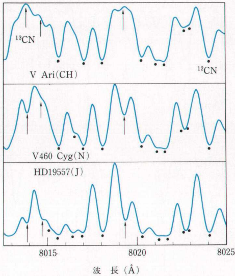
図2 CCDによる炭素星の ^{12}\text{C} N (・で示す) 及び ^{13}\text{C} N (矢印で示す)のスペクトル。ハロー種族の炭素星(CH星)の中には ^{13}\text{C} Nは見えないくらい弱く ^{12}\text{C}/^{13}\text{C} 比が 10^3 程度のものもある(上図: V Ari)が、種族Iの炭素星(N型星)では ^{13}\text{C} Nは明瞭に同定され、この例では ^{12}\text{C}/^{13}\text{C} 比は40の程度である(中図: V466 Cyg)。また、炭素星のなかには ^{13}\text{C} Nが極めて強くJ型星と分類されている炭素星があるが、その中には、 ^{12}\text{C}/^{13}\text{C} 比がCNサイクルの平衡値4以下のもの(下図: HD19557)も知られている(岡山天体物理観測所クーデ分光器による観測)。
