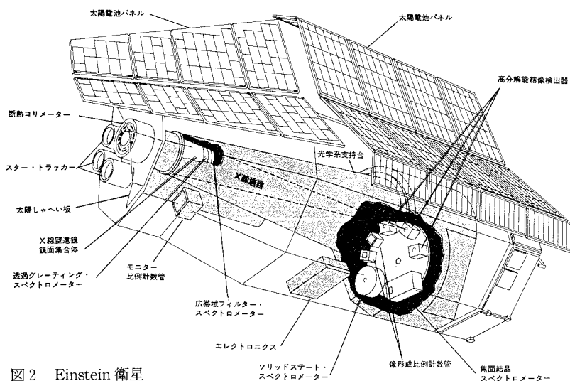
図2 Einstein衛星
