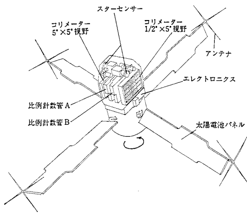
図1 Uhuru衛星
