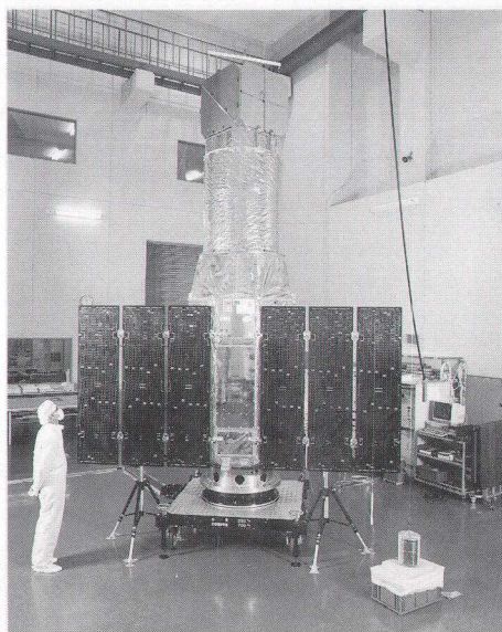
宇宙科学研究所クリーンルーム内の「あすか」。太陽電池パドルが展開し、X線望遠鏡が伸展した状態で、宇宙空間に浮かんだときとちょうど同じ姿をしている。(写真提供：文部省宇宙科学研究所)
