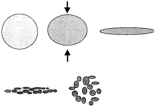
図2 パンケーキシナリオ。 先ず、大きな構造（銀河団，超銀河団）ができ、それが分裂してより小さな構造（銀河）ができていく様子を示している。
