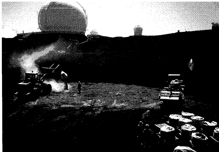
写真1 地盤改良工事：望遠鏡ピア下地盤のソイルセメント法による地盤改良は、現場の土（シンダー）にセメントと水を混ぜた後、大型の振動ローラーで転圧する。写真はセメントを改良区域に敷いているところ。向こうの大きなドームは Keck 望遠鏡。
