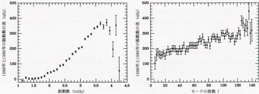
図8 太陽の音波モードの振動数の太陽活動に伴う長期変動。太陽活動が極小期に近い1986年と極大期に向かっていた1988年との振動数の差。左の図では振動数変化を振動数の関数として、右の図では l の関数としてプロットしてある。どちらの図も縦軸の単位は \text{nHz} ( =10^{-9}\text{Hz} )。Libbrecht, K. G. & Woodard, M. F. 1990, Nature , 345, 779 より転載。
