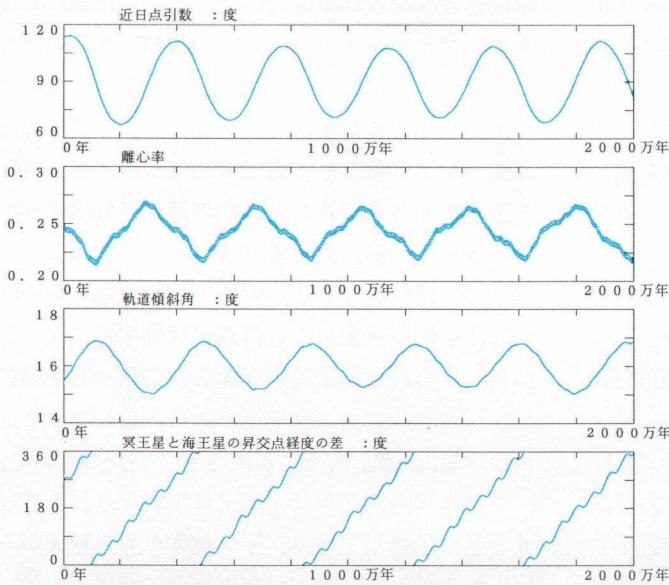
図3 冥王星の近日点指数、離心率、軌道傾斜角、冥王星と海王星の昇交点の変化。冥王星と海王星の昇交点が一致するとき冥王星の軌道傾斜角は最大、離心率は最小、近日点指数は90度となる。冥王星と海王星の昇交点の差が180度となるときには、冥王星の軌道傾斜角は最小、離心率は最大、近日点指数は90度となる。これらの変化の周期は約400万年である。
