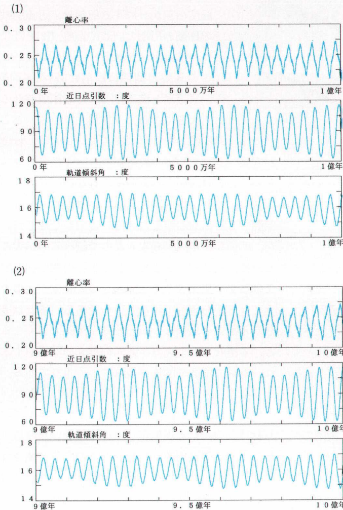
図4 (1) 現在から1億年間の冥王星の軌道要素 (2) 9億年後から1億年間の冥王星の軌道要素リアプノフ時間の40倍以上たつても軌道要素の変化には何等の不規則もみられず、非常に規則正しい。
