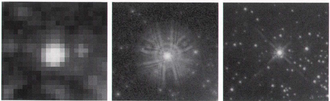
図1 大マゼラン星雲中の巨大な星形成領域にあるウォルフ・ライエ星 Melnick 34の撮像。(左)地上における約0.6秒角の星像(欧州南天天文台 G. Meylan 博士による)。(中)WF/PC-Iによる撮像。主鏡の球面収差の影響で、星の周囲に4秒角にわたる“スカート”が見える。(右)補正鏡付きのWF/PC-IIによる撮像。0.1秒角の星像を達成し、背景の暗い星の測光も可能となった。(STScI HSTNEWS より)
