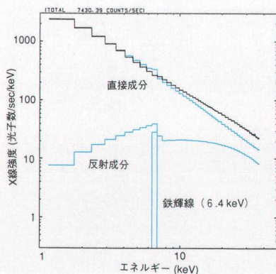
図1 ぎんが衛星が観測したCyg X-1のエネルギースペクトル。ブラックホールのまわりからやってくるべき関数成分、それが降着円盤にあたって反射された成分、中性の鉄輝線からなっている(参考文献3より)。
