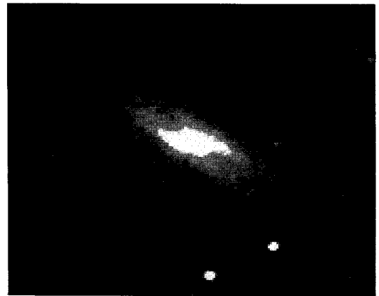
写真4 25cm反射望遠鏡で撮影したNGC253中心付近の近赤外線画像（K'バンド2.1μm）
