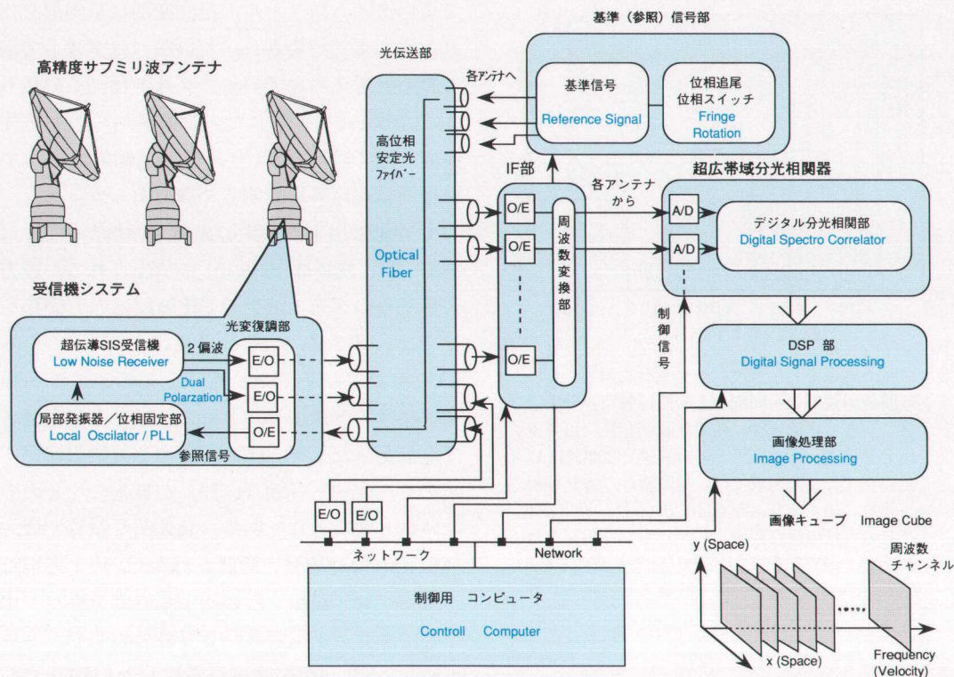
図2 LMSAの装置の概要。相互相関スペクトルを求める分光相関器には、時系列データを分光（フーリエ変換）してから相関をとるFXタイプと、相関をとってからフーリエ変換してスペクトルを求めるXFタイプがある。これらの2つの方法は、分光の方法としては等価である(Wiener-Khinchinの定理)ことが知られている。LMSAではFXタイプを採用する。DSP部は、相関器から得られたデータに対し種々の校正(遅延補正, 位相補正など)や時間積分をほどこす機能を持っている。DSP部からの信号は計算機上は蓄えられ、画像処理部で“CLEAN”法やMEM法(最大エントロピー法)を用いて電波画像に変換される。
