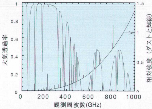
図3 大気の透過率と星形成、惑星系形成領域からの電波放射強度（星間塵からの熱輻射及び分子、原子からの輝線放射）の周波数依存性（可降水量 P.W.V.で1mm の場合の計算値）。300GHz 以上のサブミリ波領域では、星間塵からの熱輻射が非常に強くなり、350GHz、650GHz、850GHz などの大気の窓を利用して、効率よく観測を行なうことができる。LMSA では、ミリ波から850 GHz (350 \mu m) のサブミリ波帯までの観測を行なう。
