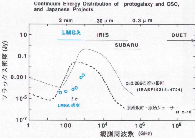
図6 予想される原始銀河，原始クエーサーの連続波スペクトル (強度の周波数依存性) と LMSA の各周波数帯での検出限界. LMSA では，銀河形成の時代 ( z=5-10 ) まで遡って，ダスト放射で明るく“輝いている”原始銀河や原始クエーサーの検出を行なうことができる. これらの遠方の天体の観測では，ミリ波からサブミリ波までカバーする LMSA は，日本の他の大型計画，IRIS (赤外線天文衛星)，SUBARU (8m 光学赤外線望遠鏡)，DUET (次期 X 線天文衛星) と相補的な関係にあり，それらの望遠鏡との協力によって，惑星系形成，銀河形成の解明に大きく近づくことができるであろう.
