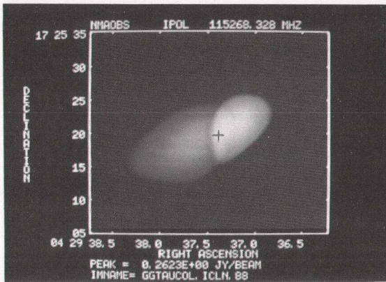
図4 野辺山ミリ波干渉計によるCOの分光観測で見いだされた若い星GG-Tau星の周りの原始惑星系円盤。太陽系の約10倍(半径500AU)で、分子ガスと塵からなり1km/sの速度で回転している。HL-Tau星で見られたような、自由落下するガスは見られず、より進化した若い星である。LMSAでは、さらに高い空間分解能、感度でもっと内側(半径10AU-100AU)の惑星系形成領域の構造に迫ることができる。
