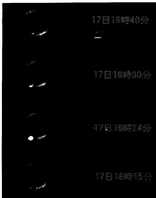
国立天文台岡山天体物理観測所188cm望遠鏡+近赤外線多目的カメラ「OASIS」によって捉えた3番目の核Cの衝突によるきのこ雲の変化。高温のきのこ雲が成長し、消滅していく様子がわかる。木星はこの波長(2.3ミクロン)では南北両極しか写らない。
