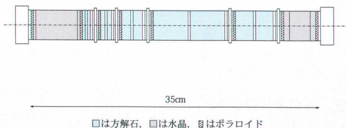
図3 磁場観測用リオー・フィルターの内部構造
