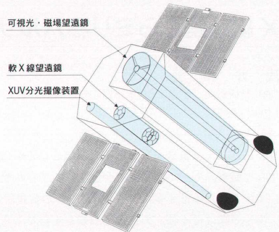
図9 計画中の太陽観測衛星
