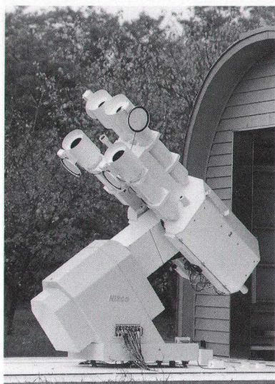
図1 国立天文台・三鷹で、ビデオ・マグネトグラフを搭載し1992年から磁場観測を行っている太陽フレア望遠鏡。
