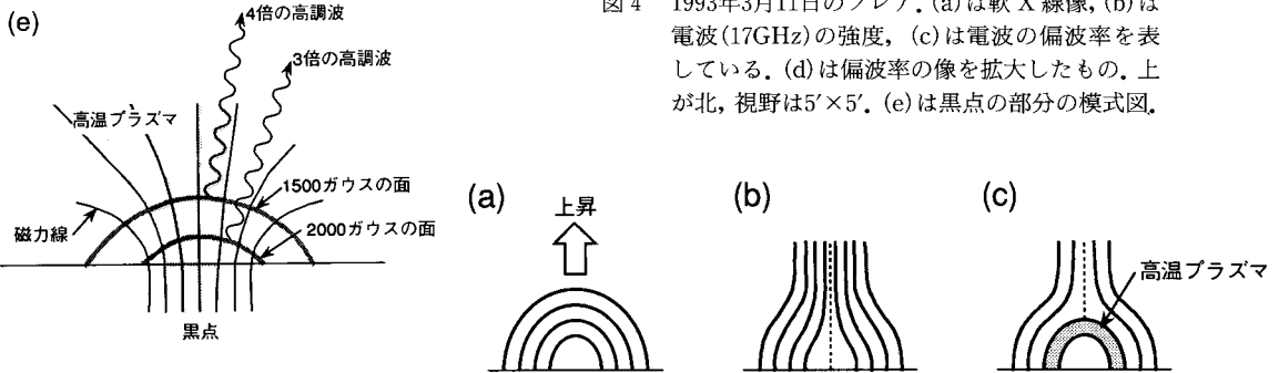
図5 Long Duration Event の模式図。閉じた磁場が上昇する 磁力線が開く 内側から順に再結合する
