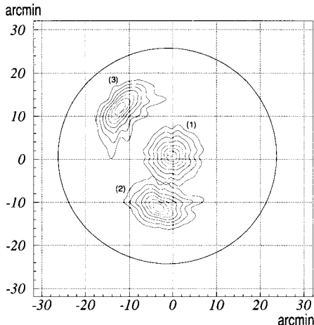
図4 「あすか」搭載のガス蛍光比例計数管による、点光源の画像の例を3つ示した。X線反射望遠鏡の特性のために、入射位置によって形が大きく変化する様子がわかる。
