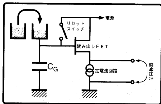
図2 CCD の出力回路
