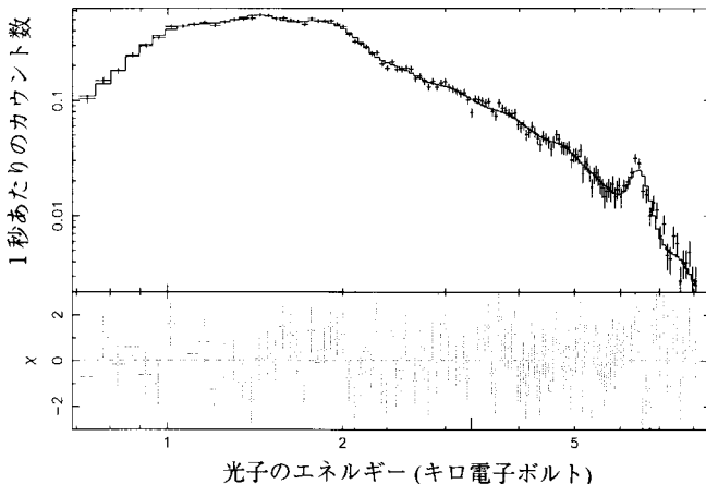
図1 「あすか」が観測した銀河団A0336+098のスペクトル。希薄なプラズマからの熱制動放射のモデルでよく説明でき、高温ガスで満ちていることがわかる。
