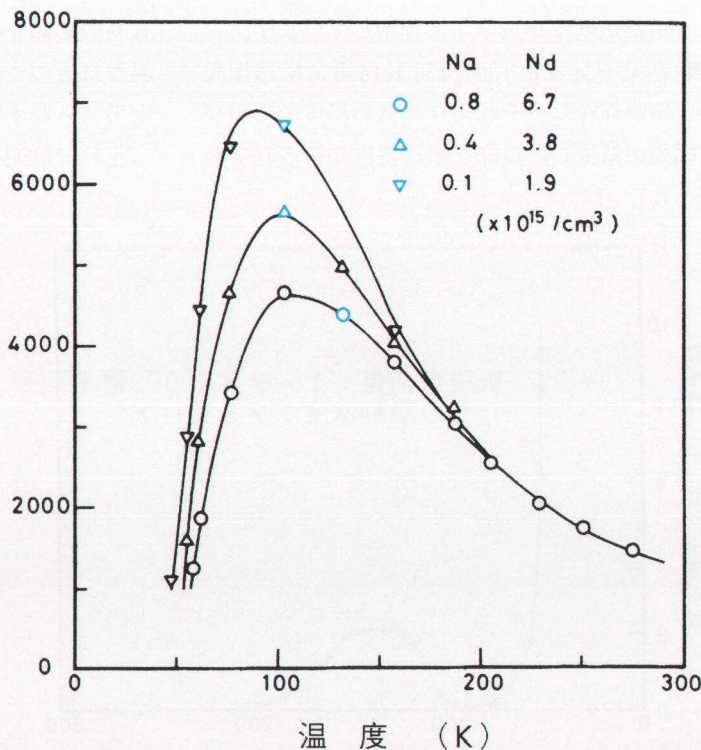
図1 電子の移動度の温度依存性
