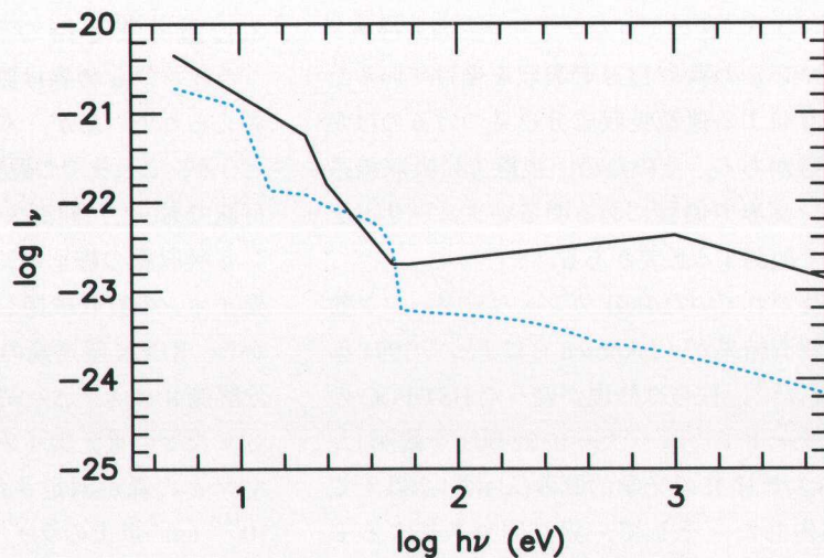
図 1 : LLS の電離状態を説明する背景紫外線輻射場の折れ曲がりスペクトル (黒線) とキューサーからの紫外線を足上げたスペクトル (青線). Denda & Ikeuchi (1995) より改 6) .
