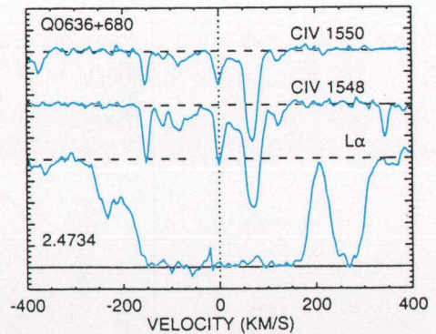
図3：ライマンαの森に付随するCIV吸収線のプロファイル例。キューサー0636+680への視線上にあるz=2.4734のライマンα吸収線（下）とCIV吸収線（上の二つ）。Cowie et al.(1995) 12) より転載。
