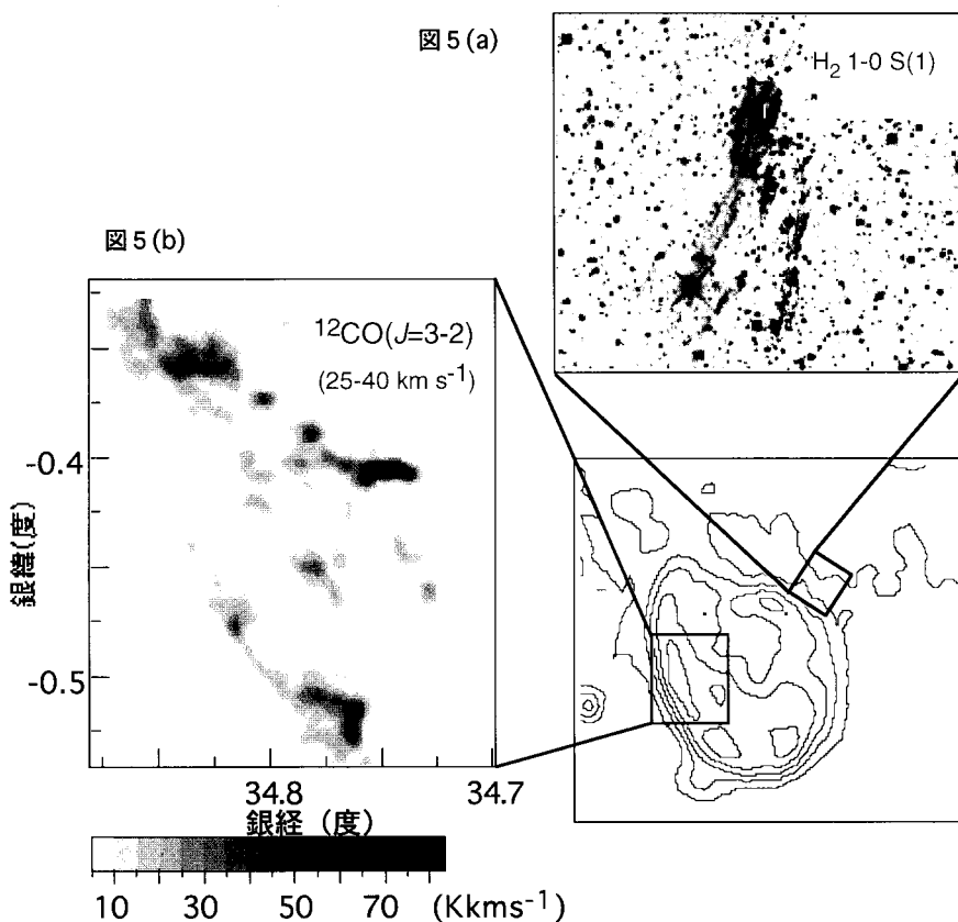
図5 (a) 岡山 188 cm 鏡による近赤外水素分子輝線 \nu=1-0 \text{ S}(1) のイメージ。連続波成分を引いていないために星が写っているが、中央部分のフィラメント状の天体が超新星残骸の衝撃波で励起された水素分子輝線である。 (b) JCMT15 m 鏡による ^{12}\text{CO} (J=3-2) 輝線観測で浮かび上がったショックガス。
