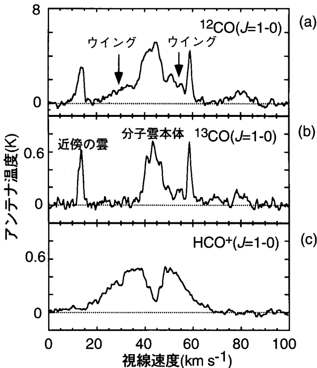
図4 (銀経, 銀緯)=(34.75度, -0.40度)におけるスペクトル。(a) ^{12}\text{CO} , 40\text{ km s}^{-1} の分子雲本体からウイングが延びている。(b) ^{13}\text{CO} , 分子雲本体の成分のみが見える。(c) \text{HCO}^+ , 分子雲本体に対応する速度における窪みは自己吸収である。線幅 60\text{ km s}^{-1} にわたる加速されたガスが明瞭に見えている。
