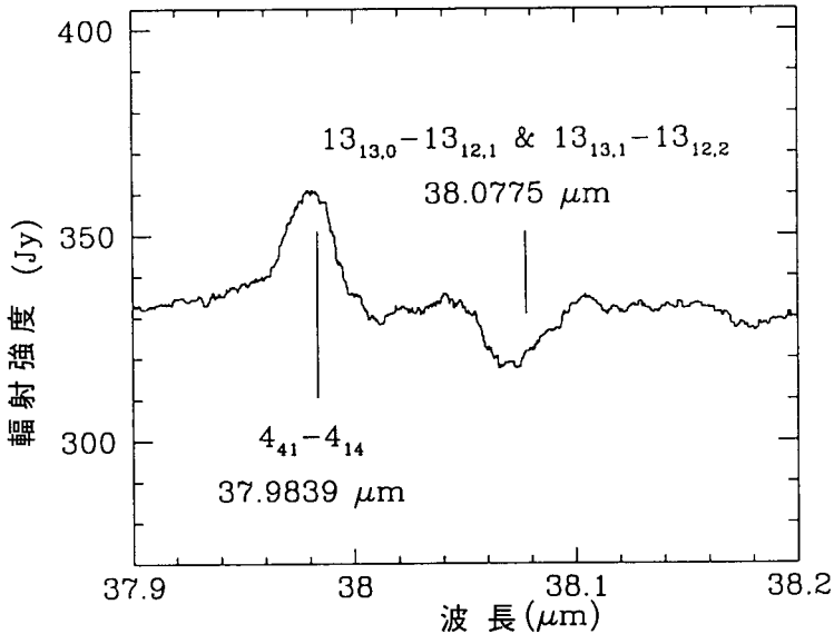
図3. 水 ( \text{H}_2\text{O} ) 分子の遠赤外線 8)
