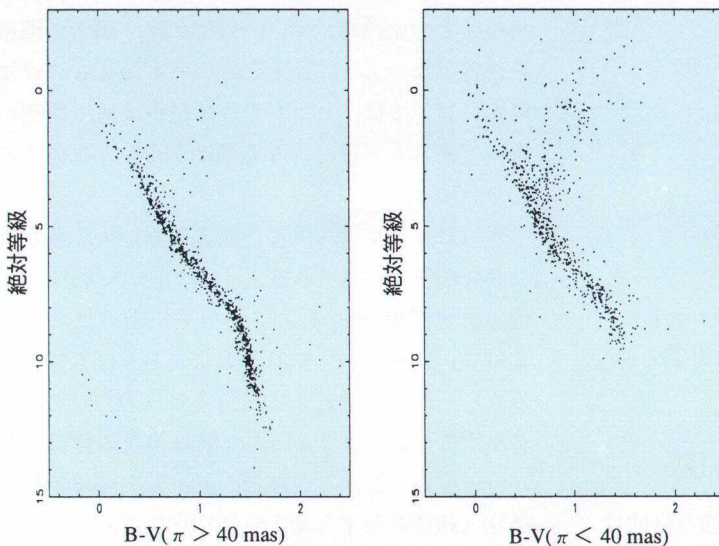
図3 ヒッパルコス視差に基づくグリーゼ星表星のH-R図
