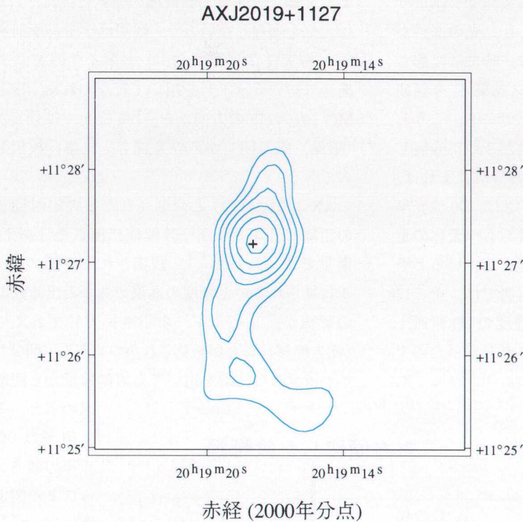
図3：ドイツのX線天文衛星「ローサット」のHRI（高分解能撮像装置）によって観測された銀河団 AX J2019+1127 のX線像。等高線はX線強度を表す。強度最大の点は中心銀河（十字点）とほぼ一致している。X線像は広がっていて、赤方偏移 z=1 における我々の銀河の数千倍の質量を持つ銀河団の大きさとも一致する。
