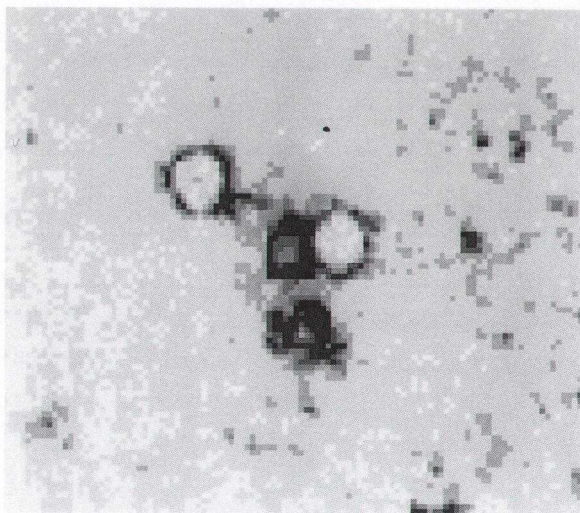
図 1 : MG2016+112 の可視光像(疑似カラー) 2つの白い丸がレンズされたクェーサー。3.4 秒角離れている。右の白丸のすぐ左にある黒い天体が、赤方偏移 z=1 にあるレンズ銀河。この銀河と同じ z の所に X 線銀河団が発見された。下の黒い天体は偶然手前にある銀河。クェーサーの 3 つめの像は、その銀河と重なっている。
