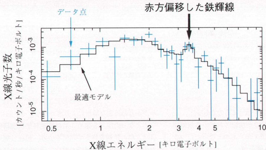
図2：「あすか」の GIS 検出器(位置検出型ガス蛍光比例計数管)によって観測された銀河団 AX J2019+1127 の X 線スペクトル。温度 1 億度(10 8 K)のほぼ太陽組成のプラズマからの熱 X 線放射モデルで良く合っている。この温度から、この銀河団の重力質量は、我々の銀河の数千倍と考えられる。太矢印は赤方偏移した鉄原子の輝線。静止系でのエネルギーは 6.7 キロ電子ボルトと 6.9 キロ電子ボルトである。これより赤方偏移量 z が求められ、それは、重力レンズ効果から予測されていたもの ( z=1 ) にほぼ一致する。
