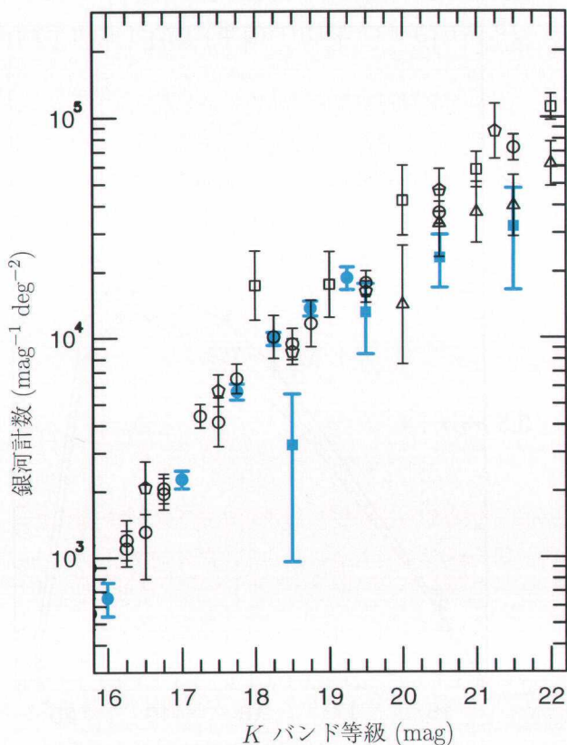
図5 われわれの観測から得られた銀河計数と他の観測との比較。青丸が the bright survey を、青四角が the faint survey を示しています。K = 17–19 mag で the bright survey の誤差がもっとも小さいことがわかります。
