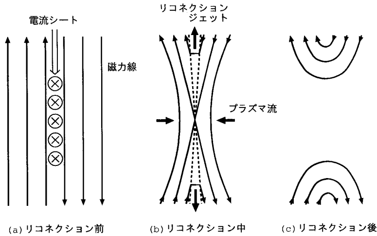
図3 磁気リコネクションの概念図。(a) 反平行の磁力線が接触している状態。磁気中性面に電流が流れ(電流シート), そこでは電気抵抗により磁力線が消失する(拡散領域)。(b) 拡散領域で磁力線のつながりかえ(磁気リコネクション)が起こり, 磁気張力により磁力線が図の上下にはじけとんでいく。この上下の流れはリコネクション・ジェットと呼ばれ, アルファベン速度程度の速さである。(c) 磁気リコネクションにより, 磁力線のつながり方が(a)と変わる。
