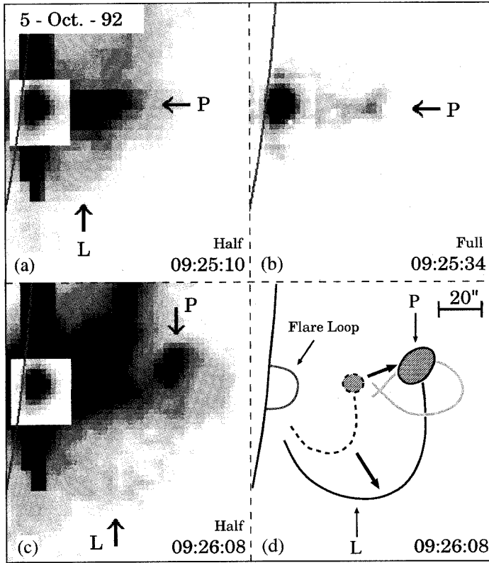
図7 軟X線で観測された1992年10月5日のフレアに伴うX線放出プラズマの時間変化. 図5と比べ広視野で露出時間が長い(a: 78ミリ秒, c: 38ミリ秒). (b)は図6の画像. (d)は(c)の概略図を表し, 点線は(a)での放出プラズマを示す. これらの図から, 放出プラズマは塊状のプラズマ(いわゆるプラズモイド)だけでなく, ループ構造も含んでいることが分かる. (大山と柴田 9) より)
