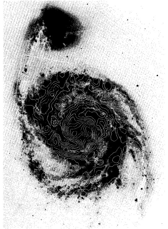
図1. 光学写真(白黒反転)に重ねたM51のCO積分強度図 1) 。白い枠が観測した範囲。
