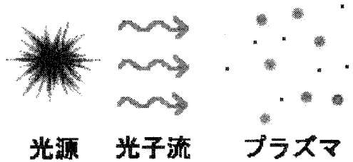
図2 a 輻射圧
