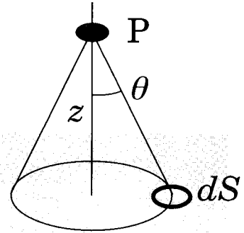
図4 平面光源
