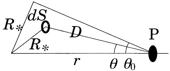
図3 球状光源
