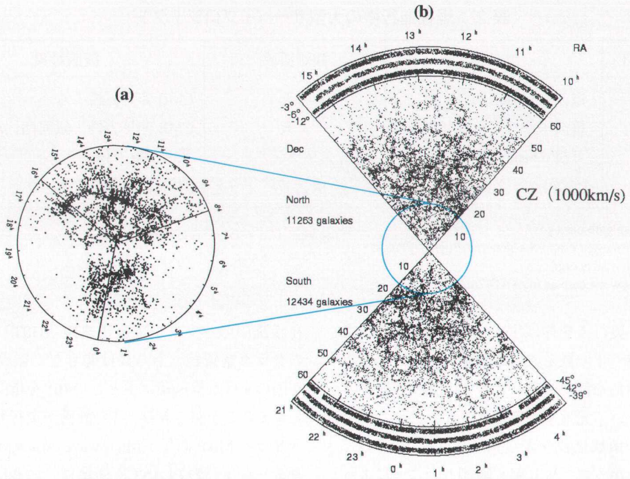
図1 銀河サーベイの進化：(a) CfA サーベイ 11) , (b) Las Campanas Redshift Survey 12) .
