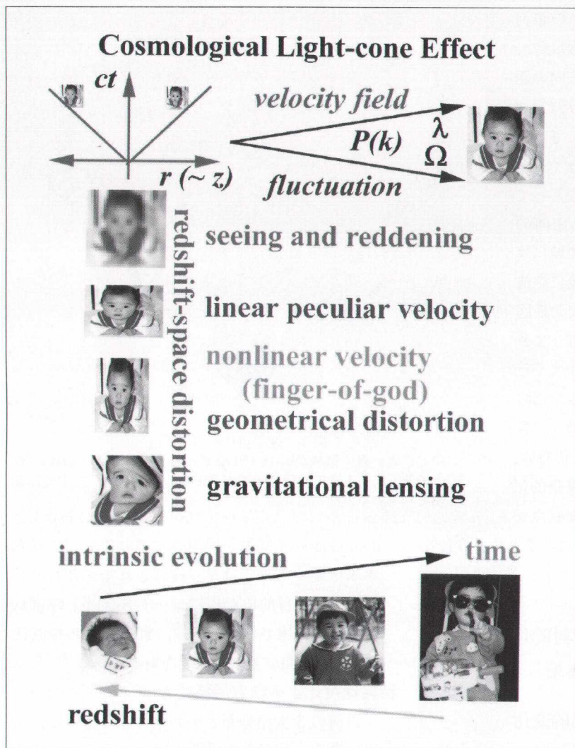
図4 宇宙論的観測にともなう困難。
