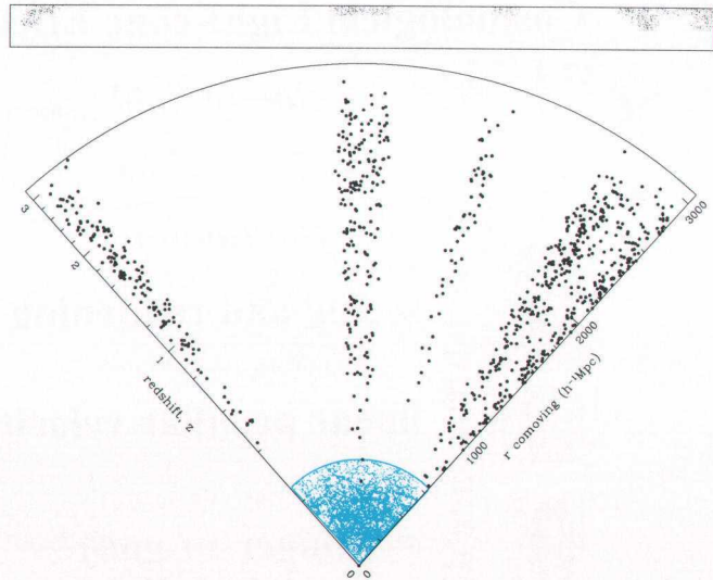
図3 遠宇宙サーベイ 中心に近い青い領域が図1bのLas Campanas Redshift Survey 12) の下半分. Z = 3 までのびた領域が2dF Quasar Survey 14) ですでに観測されている分布.
