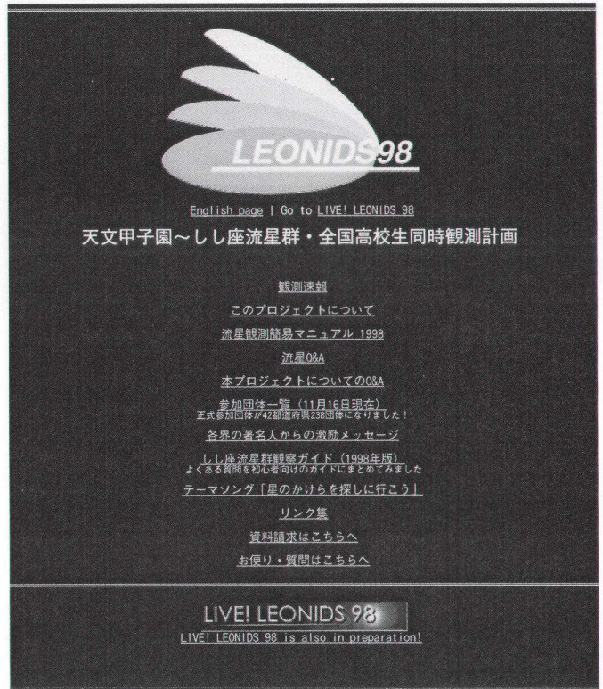
図1：しし座流星群全国高校生同時観測会ホームページ ( http://www.leonids.net/ )
