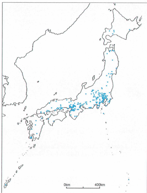
図2：観測に成功した全国208箇所の観測点 作成：小川宏，山本雅之
