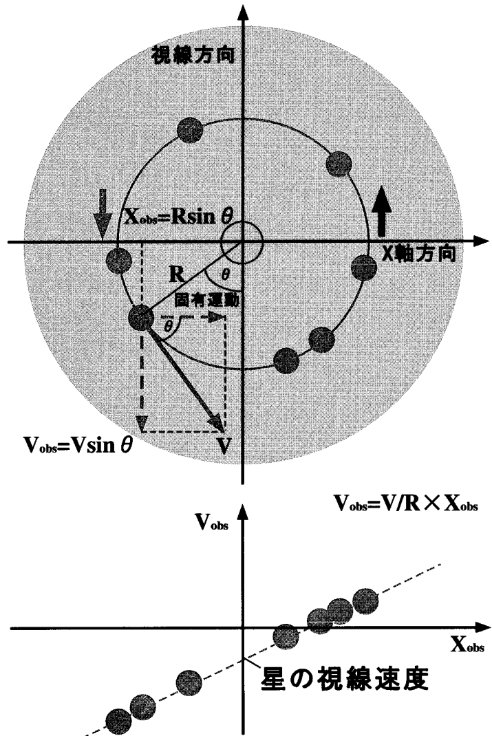
図2：上図) 回転ガス円盤とその上で中心星の周りを回転運動するメーザースポットを真上から見たときの、メーザースポットの位置と運動方向の関係。下図) 円盤上の同一半径円上で回転運動するメーザースポット群を、エッジオンで(円盤面を横から)見た時に得られる、メーザースポット群の位置・視線速度図。
