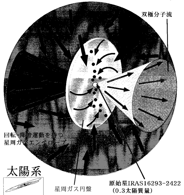
図4：原始星 IRAS 16293-2422 (A)を取り巻く、回転ガス円盤、星周ガスエンベロープ、双極分子流の想像図。
