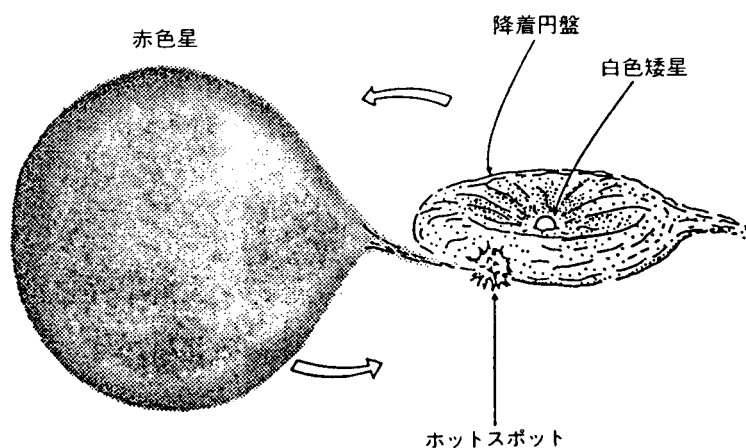
図2. 激変星近接連星と降着円盤 22) . 激変星は、白色矮星と赤色星との半分離型近接連星である。ロッシュ限界を満した赤色星からガスが流出し、白色矮星のまわりに降着円盤を作る。赤色星から流出したガスが降着円盤と衝突する場所に衝撃波面が出現、明るく輝く。そこをホットスポットと呼ぶ。
