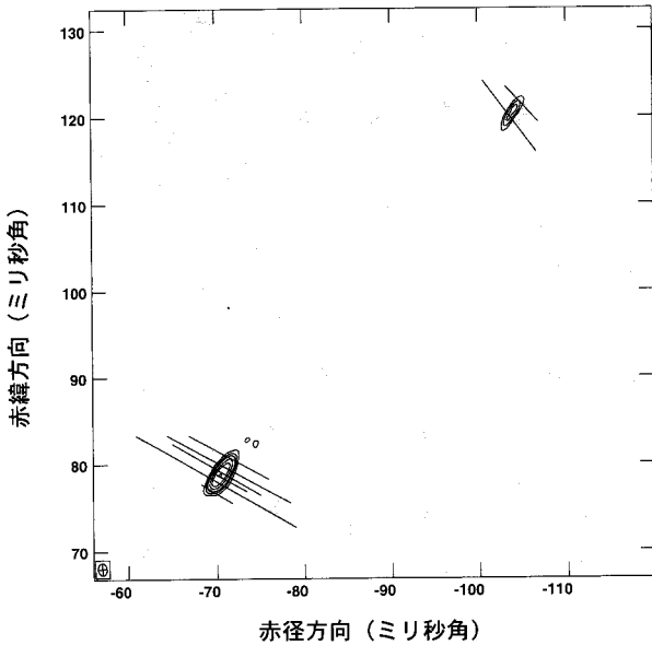
図2 オリオン KL 領域の隣接する水メーザースポットの偏波構造の例 (堀内ら 8) による 1997 年 2 月の VLBA 観測結果から). 星間空間の水メーザーはヒモ状に分布することが多いが, このオリオン KL 領域の観測により隣り合うスポットの偏波プロファイルは似ていることが多いことがわかった. このことはメーザースポットが大局的な磁場に支配されていることを強く示唆している. 図は電波源 I から南西に約 6 秒角 (約 3000AU) ほど離れたメーザースポットのマップで, コントアはトータル強度, コントア上の棒線の長さ, 角度がそれぞれメーザー放射の直線偏波率, 偏波角をあらわす. トータル強度は 30 ジャンスキー以下と, この領域のメーザーには極めて微弱ながら, 偏波率はいずれも約 70% ほどで, 二つのうち下のスポットが, この観測の 10 ヶ月後にメーザーバースト現象を起したことが, バースト中の VLBI 観測との比較でわかった. メーザースポットの並びが図 1 の円すい形フローと同様, ラージスケール的高速双極分子流の方向と平行であることに注意.
