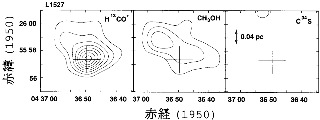
図4 L1527 領域における \text{H}^{13}\text{CO}^+ ( J = 1-0 ) (左), \text{CH}_3\text{OH} ( J_K = 2_0-1_0 A^+ ) (中央), \text{C}^{34}\text{S} ( J = 2-1 ) (右) 輝線の積分強度図 ( 5.2-7.3 \text{ km s}^{-1} ). コントアレベルは 0.12 \text{ K km s}^{-1} から 0.08 \text{ K km s}^{-1} おき. 十印は原始星 IRAS 04368+2557 の位置を表す.
