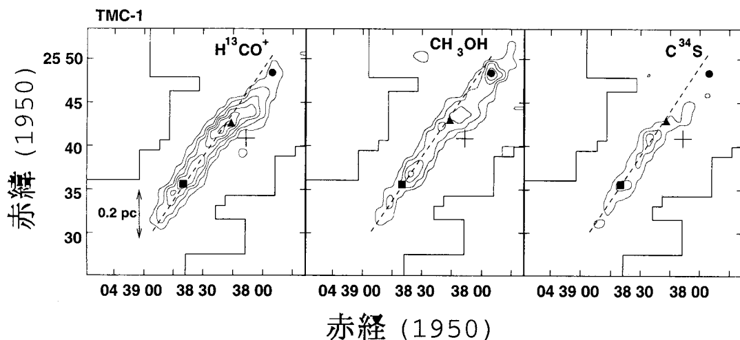
図2 TMC-1 領域における H^{13}CO^+ ( J=1-0 ) (左), CH_3OH ( J_K=2_0-1_0 A^+ ) (中央), C^{34}S ( J=2-1 ) (右) 輝線の積分強度図. ( 5.6-6.4 \text{ km s}^{-1} ). コントアレベルは 0.10 \text{ K km s}^{-1} から 0.08 \text{ K km s}^{-1} おき. 十印は原始星 IRAS 04381 + 2540, ■はシアノポリンピーク, ▲はアンモニアピーク, ●は TMC-1 CH_3OH の位置を表す. 破線は図3の位置—速度図の切った線を表す.
