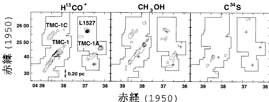
図1 おうし座分子雲における H^{13}CO^+ ( J=1-0 ) (左), CH_3OH ( J_K=2_0-1_0 A^+ ) (中央), C^{34}S ( J=2-1 ) (右) 輝線の積分強度図 ( 4.8-7.2 \text{ km s}^{-1} ). コントアレベルは 0.20 \text{ K km s}^{-1} から 0.10 \text{ K km s}^{-1} おき. 十印は原始星の位置を表す.
