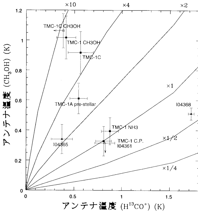
図6 おうし座分子雲中の9つの場所における H^{13}CO^+ 輝線と CH_3OH 輝線の強度相関図。エラーバーは 1\sigma 。矢印のついたプロットは 3\sigma の上限を表す。四角のマークは原始星の付随しない場所、三角のマークは原始星の付随する場所における強度相関を表す。複数のカーブはLVGモデルで計算した強度相関。それぞれのカーブは、 H^{13}CO^+ に対する CH_3OH の相対的な存在量が \times 1 , \times 2 , \times 4 , \times 10 , \times 1/2 , \times 1/4 の場合を表す。
