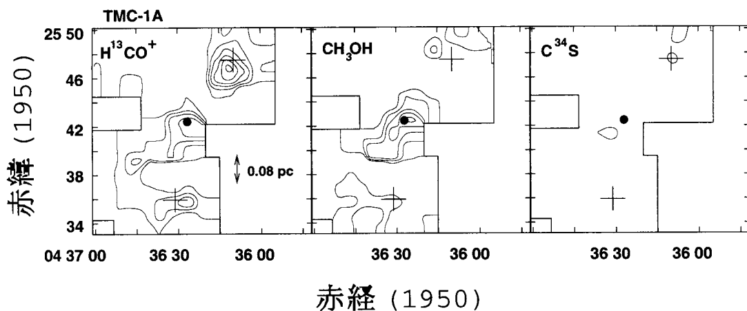
図5 TMC-1A 領域における \text{H}^{13}\text{CO}^+ ( J=1-0 ) (左), \text{CH}_3\text{OH} ( J_K=2_0-1_0 A^+ ) (中央), \text{C}^{34}\text{S} ( J=2-1 ) (右) 輝線の積分強度図 ( 6.1-6.9 \text{ km s}^{-1} ). コントアレベルは 0.10 \text{ K km s}^{-1} から 0.05 \text{ K km s}^{-1} おき. 十印は原始星, ●印は TMC-1A pre-stellar の位置を表す.
