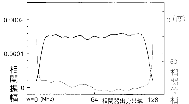
図5：受信機1にレンズ素片をかざしたときの相関器出力： S(w)_0 の振幅と位相
