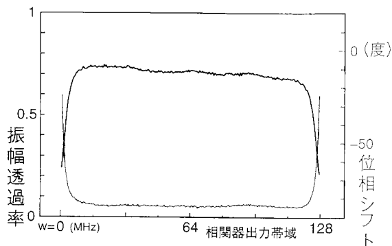
図7: レンズ素片の透過率: \text{abs}(\frac{S(w)_i}{S(w)_o}) と 位相シフト量: \text{arg}(\frac{S(w)_i}{S(w)_o})
