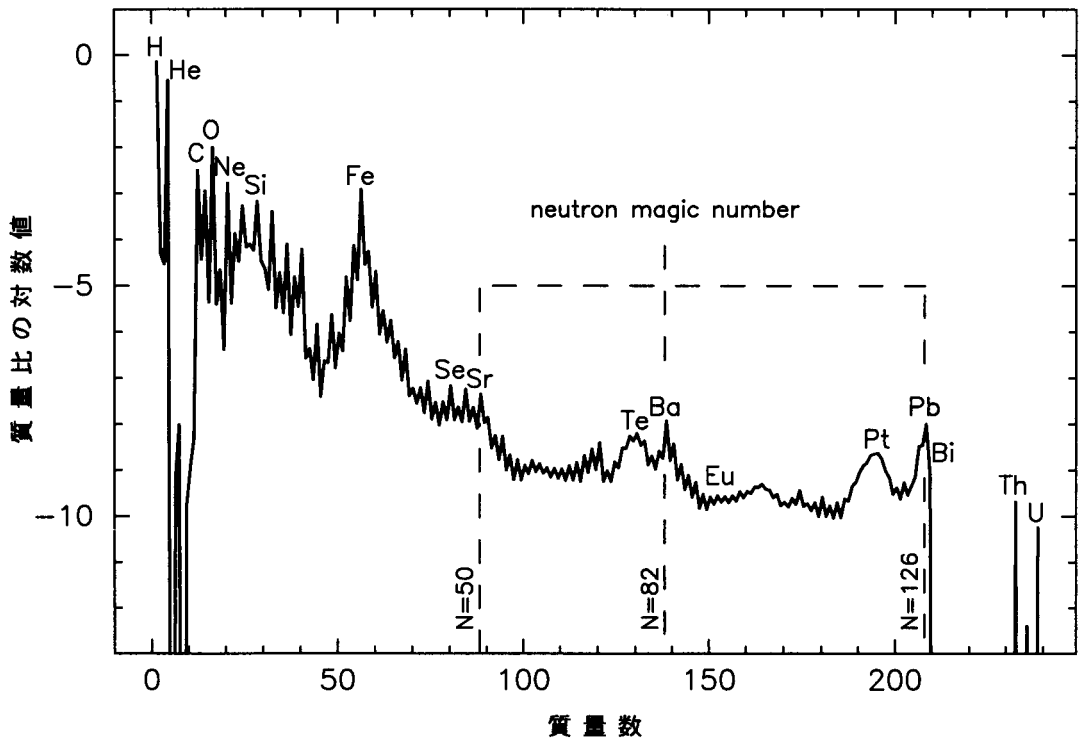
図1 太陽系の元素組成比 1) 。鉄より重い元素組成比は、中性子のマジックナンバー 50, 82, 126 とその少し手前にピークをもつ。
