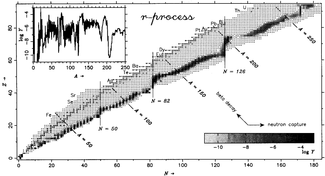
図5 ダイナミック r プロセスによる元素合成の計算例 6) 。横軸は中性子数、縦軸は原子番号。点は原子核反応ネットワークに組み込まれている核種で、中性子、陽子からプルトニウムまでの3000個以上におよぶ。青点は、安定核および長寿命放射性元素を表す。グレイスケールは、中性子捕獲反応が凍結したときの核種の存在量を表す。左上には、その対数値を質量数の関数として表してある。中性子のマジックナンバー付近にピークを作っているのがわかる。これらはこの後ベータ崩壊によって安定核へ向かうため、ピーク位置はマジックナンバーより少し手前にシフトする。
