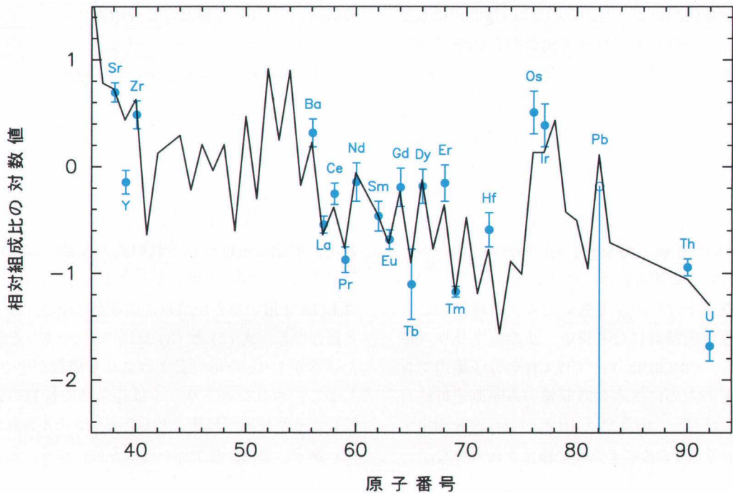
図4 超金属欠乏星 CS31082-001 の重元素パターン (青円) 16) 。鉛 (Pb) については上限値を示す。実線は太陽系 r プロセス元素パターン。原子番号 56 以上 72 以下では太陽系 r プロセスとはほぼ一致しているが、r プロセスの第 3 ピーク付近 (Os, Ir) では明らかに異なる。
