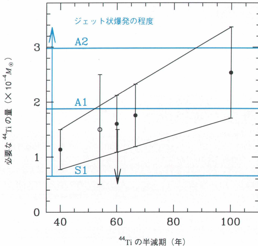
図2 爆発後3600日のボロメトリックな光度を説明するために必要な ^{44}\text{Ti} の量。横軸は ^{44}\text{Ti} の半減期。四角で囲った領域は Mochizuki et al.1999 による 25) 。白丸はBバンドやVバンドの光度を使って求めた ^{44}\text{Ti} の量 26) 。矢印はFe 25.99 \mu\text{m} のフラックスから求めた上限値 27) 。S1, A1, A2は著者の計算による元素合成の計算結果。S1は球対称爆発モデル, A1, A2はジェット状爆発モデルで、極と赤道に於ける速度比がそれぞれ2:1と4:1に対応する。 ^{44}\text{Ti} の半減期は最近の実験で60年程度とほぼ確定しており 43) 、A1モデル程度のジェット度合が適当と思われる。尚、 ^{56}\text{Co} 、 ^{57}\text{Co} の量は全てのモデルで観測量を再現している 29) 。
