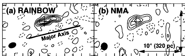
図4：NGC 3628 の 3 mm 連続波の画像。中心のクロスは VLA で測定されたセンチ波連続波のピークであり、本観測の視野中心である。等高線はノイズレベルの 1.5 倍毎に引いている。左下の黒丸はビームサイズである。(a) RAINBOW のデータから作った画像。ビームサイズは 1.8 \times 1.2 秒。ノイズレベルは 0.55 mJy。(b) NMA (左のデータから 45 m 鏡のデータを引いたもの) のデータから作った画像。ビームサイズは 1.7 \times 1.5 秒。ノイズレベルは 0.75 mJy。
