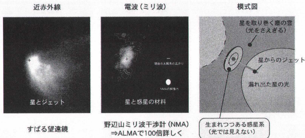
図4 おうし座暗黒星雲内の原始星 L1551 IRS5 の、『すばる』による近赤外線画像 4) と、野辺山ミリ波干渉計が描き出した C 18 O J=1-0 ミリ波輝線によるイメージ 5) 。近赤外線では、原始星のジェットと、双極流によって作られた空洞からもれ出す原始星の光が見えるのに対して、ミリ波では星を取り巻く原始惑星系円盤が見える。ALMA によれば、100 倍の分解能でその詳細な構造と運動を調べることができる。(国立天文台 提供)
