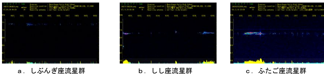
図-1 各流星群の代表的なHROFFT画像
