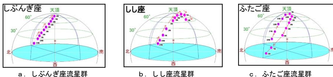
図-2 各流星群の輻射点の日周運動
