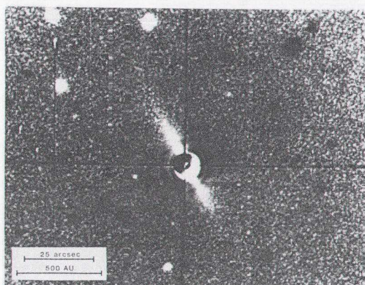
図1 がが座ベータ星で見つかった塵円盤。中央の十字でがが座ベータ星自体を隠している。
