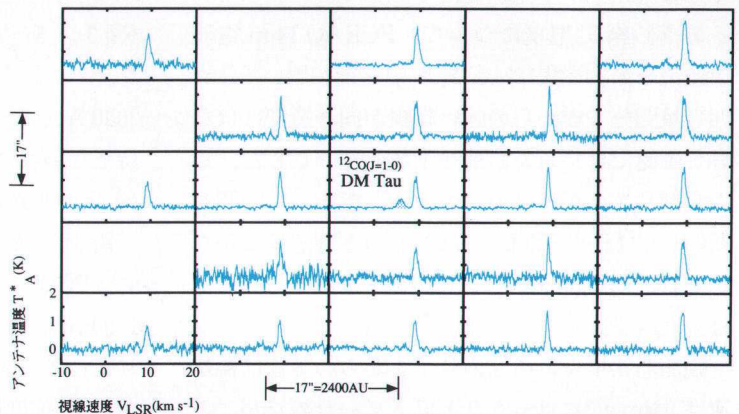
図3 おうし座DM星周りのCO輝線の様子。1つずつの枠の間隔は17秒角。おうし座分子雲の距離では2400AUに相当する。おうし座DM星の方向は図の中央。水色に塗られた輝線は中心の枠でのみ見られることから、おうし座DM星に付随していると推定される。
