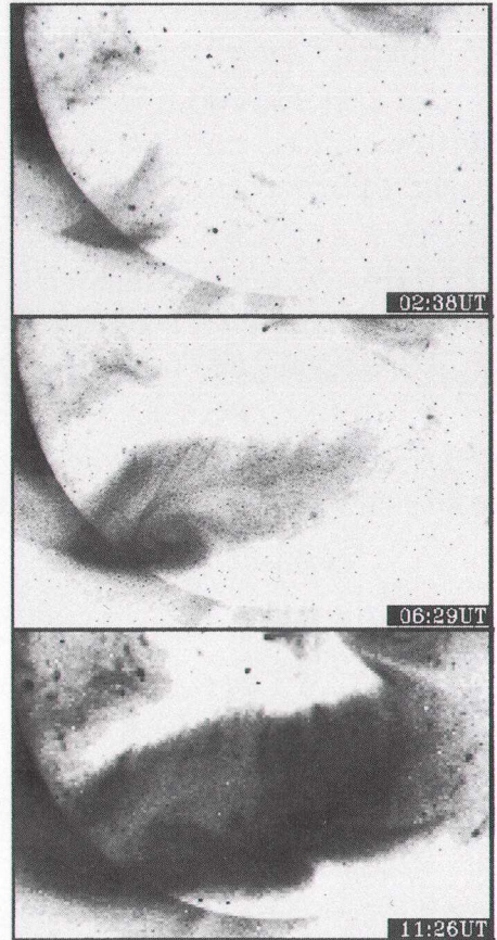
図7 「ようこう」軟X線望遠鏡で観測された1994年4月14日の巨大アーケード(McAllister他11)。図はネガ。コロナ質量放出にともなって発生した。リコネクションを示唆するカスプ構造がはっきり見え、長寿命(LDE)フレアの形にそっくりである。2日後に巨大磁気嵐が地球で発生したが、「ようこう」観測に基づく予報のおかげでアメリカ・シカゴの電力会社が変圧器(これだけで5~10億円かかるという)などの破損の被害をまぬがれた。
