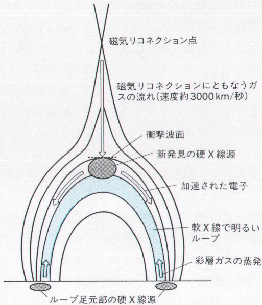
図6 インパルシブ・フレアのリコネクション・モデル (増田他 8) )。軟X線ループの上空に発見された硬X線源は、ループの上空で磁気リコネクションが起きていることを示唆する。すなわち、リコネクションにともなうガスの流れ(リコネクション・ジェット=速度約3000km/s)がループに衝突したところに衝撃波が発生して、新発見の硬X線源を形成すると思われる。
