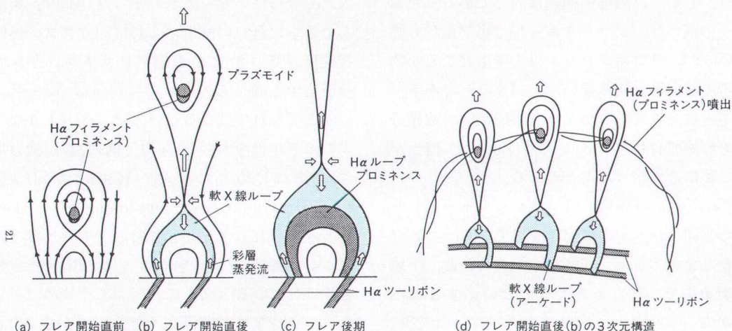
図4 フレアのCSHKP-リコネクションモデル (柴田・小杉 1) より)。大規模磁気ループの膨張とともに低温プラズマ (H \alpha プロミネンス) または高温プラズマ (しばしばプラズマモイドと呼ばれる) の噴出がある。このモデルは Carmichael, Sturrock, Hirayama 6) , Kopp and Pneuman といった人々によって発展させられた。それゆえ CSHKP モデルと呼ばれる。
