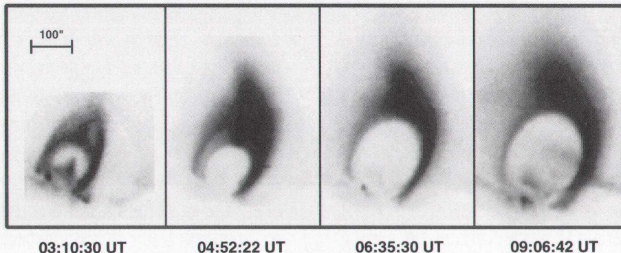
図3 軟X線 (1 keV 程度) で見た長寿命 (LDE) フレア (1992年2月21日のフレア; 常田ら 4)5) の時間変化。時間とともにカスパ型ループは次第に大きくなる。これは見かけ上の運動である。図はネガ。100''は約72000km に対応。
