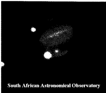
‘PANIC’がとらえた SL-9H 核の木星表面衝突、G 核の衝突跡と木星の衛星イオとガニメデも見える。
