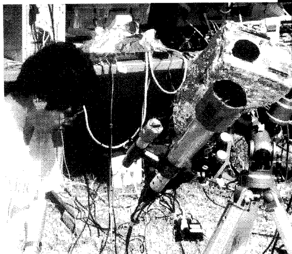
図8 アルミホイルで作成したボックス内に分光器が入っている。
