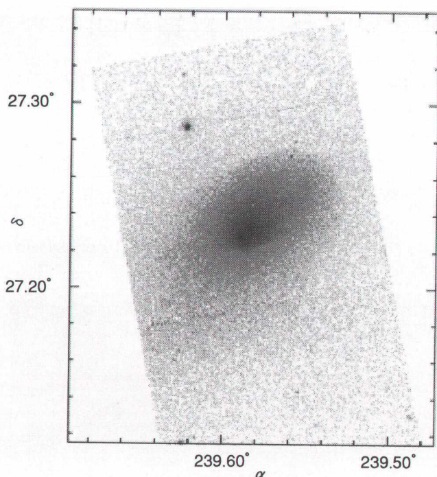
図1 チャンドラで撮影した銀河団 Abell 2142 の中心部。黒いところがX線で明るいところ。
